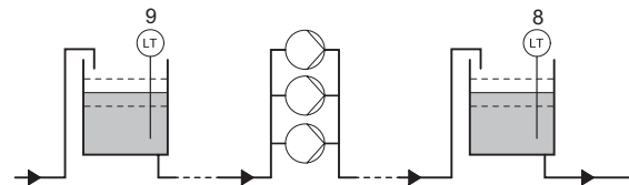
7-сур. Деңгейін бақылау
