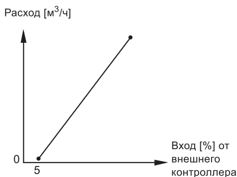
Рис. 27 Регулировочная характеристика для разомкнутого контура
