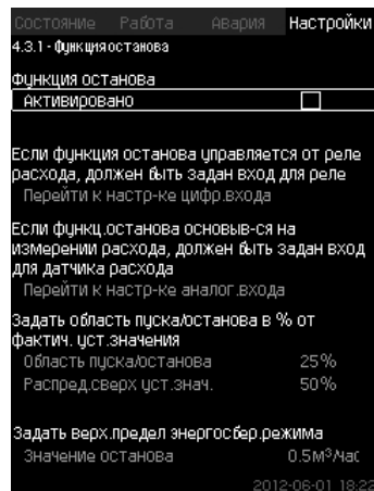
Рис. 67 Функция останова
