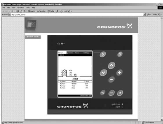
Рис. 124 Настройки сети
