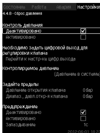
Рис. 107 Сброс давления
