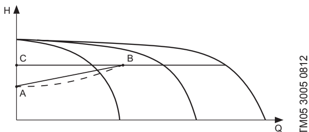
Рис. 51 Пропорц. давление
