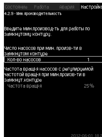
Рис. 64 Мин. производительность
