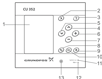
Рис. 8 Панель управления
